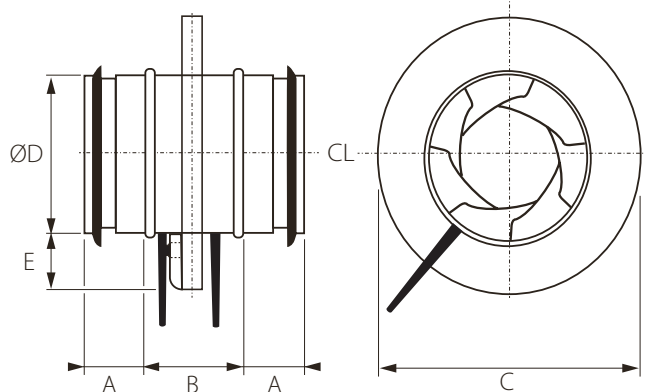
Bild 1. Mått (mm).
