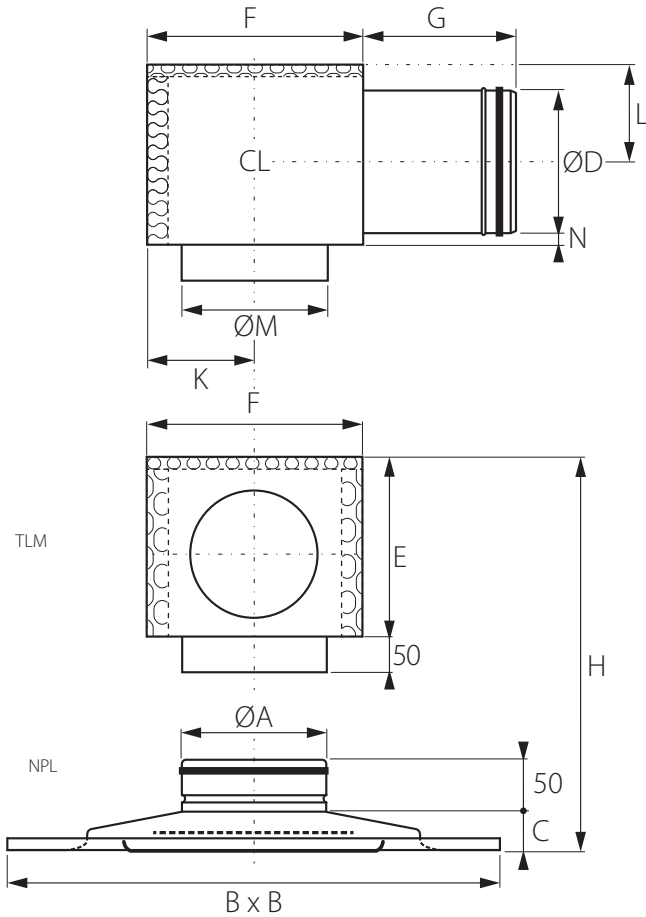
Billede 3. Målskitse (mm), Loftdiffuser NPL og trykfordelingsboks TLM.
