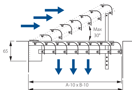
Bild 3. Mått (mm), luftriktarspjäll LS.
