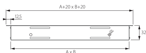
Bild 1. Mått (mm), fästram RAM.
