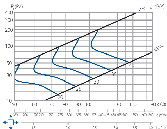
D4: NHL-M Ø200 – TLM Ø200-200
