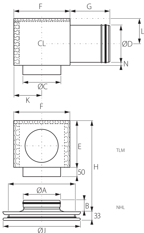
Billede 3. Målskitse (mm), Loftdiffuser NHL og trykfordelingsboks TLM.
