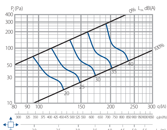
D6: NHL-M Ø250 – TLM Ø250-250
