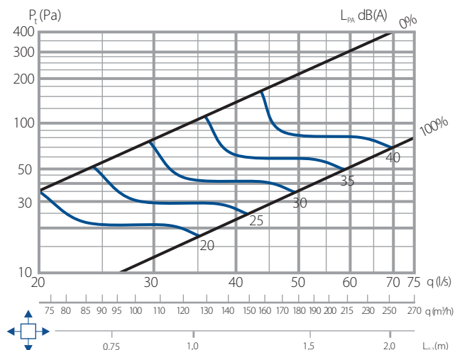
D1: NHL-M Ø160 – TLM Ø160-125
