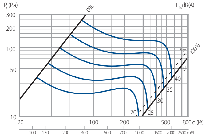
D13: FLKR Ø400 + E5 600-300
