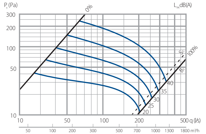
D12: FLKR Ø315 + E5 600-200
